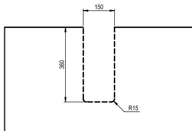
SCANSO SUL TOP PER CONSOLLE TWENTY IN APPOGGIO
