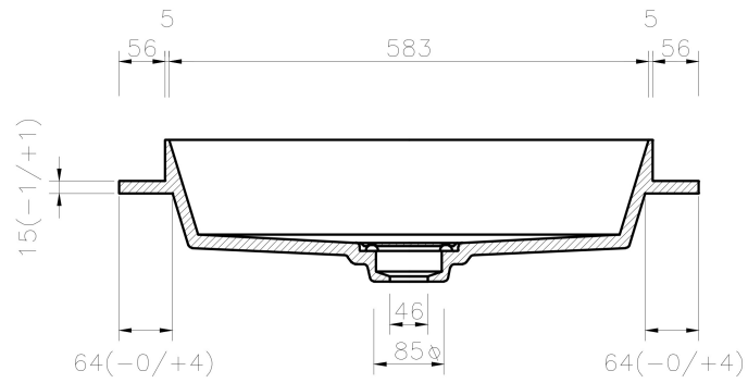
SEZIONE A-A SCALA 1:10
