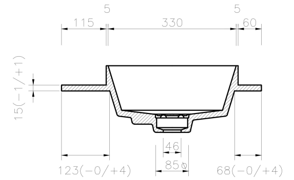
SEZIONE B-B SCALA 1:10
