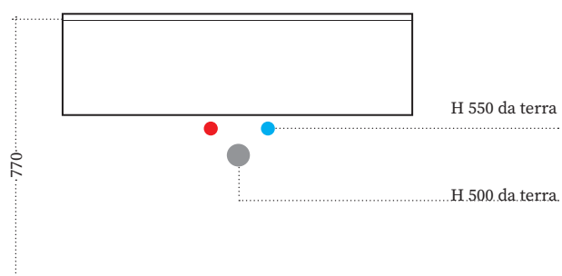
BASI 60 - 80 con top in appoggio
