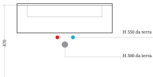
BASI 60 - 80 con vasca integrale
