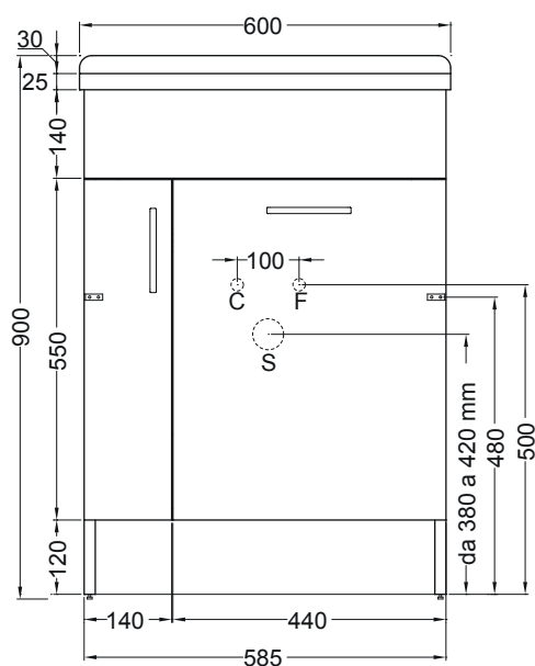
VISTA FRONTALE
