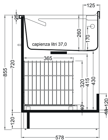
SEZIONE A-A'
