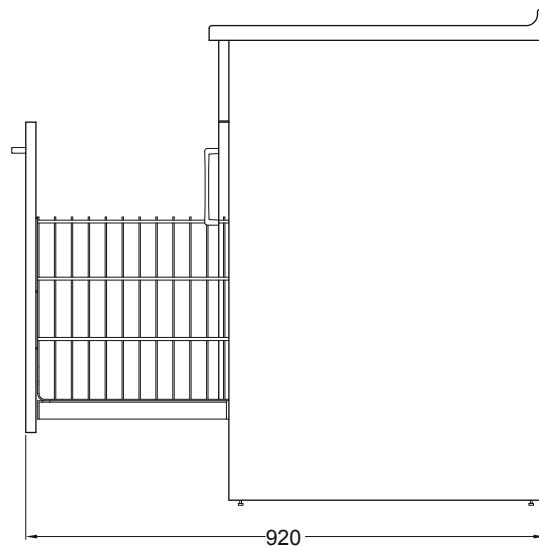
VISTA LATERALE CON CESTO APERTO
