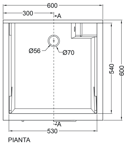
PIANTA
