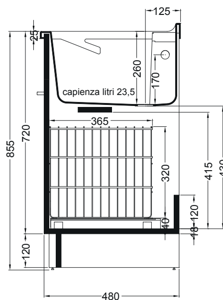
SEZIONE A-A'
