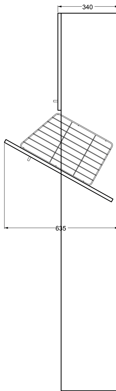
VISTA LATERALE
