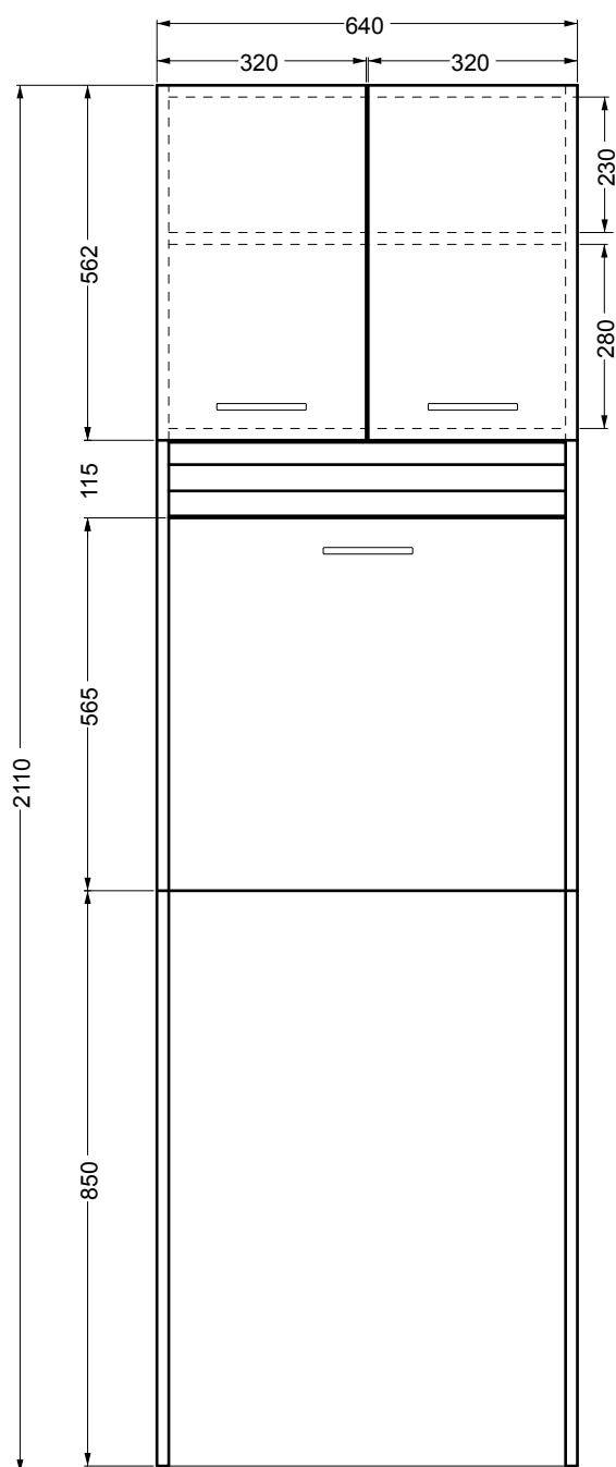
VISTA FRONTALE
