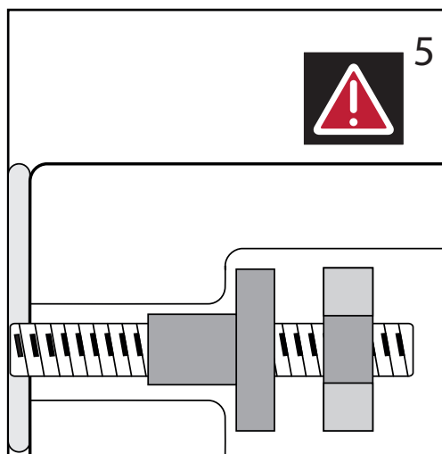
FIG5 FARE ATTENZIONE, TRA IL DADO IN METALLO E LA CERAMICA, INSERIRE L'APPOSITA RONDELLA IN PLASTICA COME DA DISEGNO WARNING: INSERT A WASHER BETWEEN THE METAL NUT AND THE CERAMIC PRODUCT AS SHOWN IN THE PICTURE
