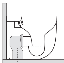
180 mm con curva art. 900102
