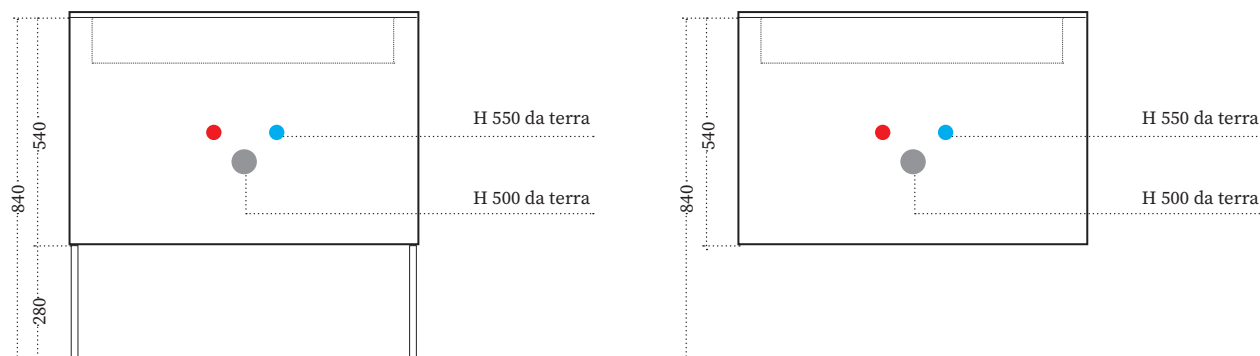
BASI 70 / 90 - con incasso o semi incasso
