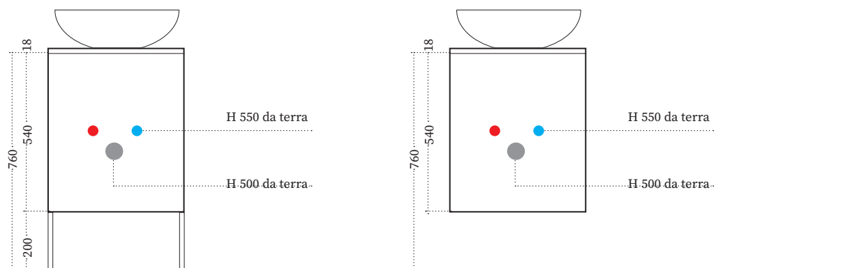
BASE 50 - con vasca in appoggio
