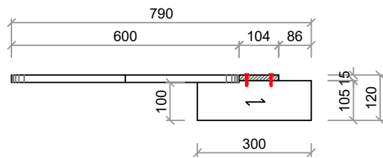
TOP VIEW T. Atas
