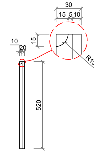
T. SAMPING PINTU SCALE 1:10
