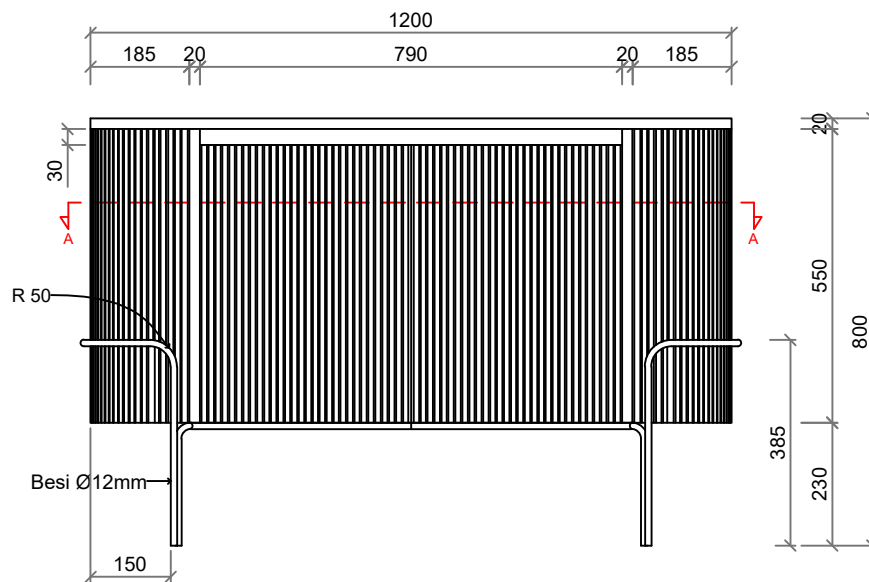
T. DEPAN SCALE 1:10
