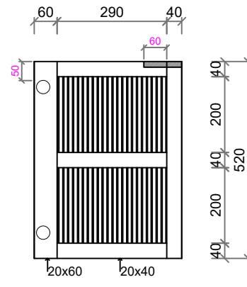
T. BELAKANG PINTU SCALE 1:10
