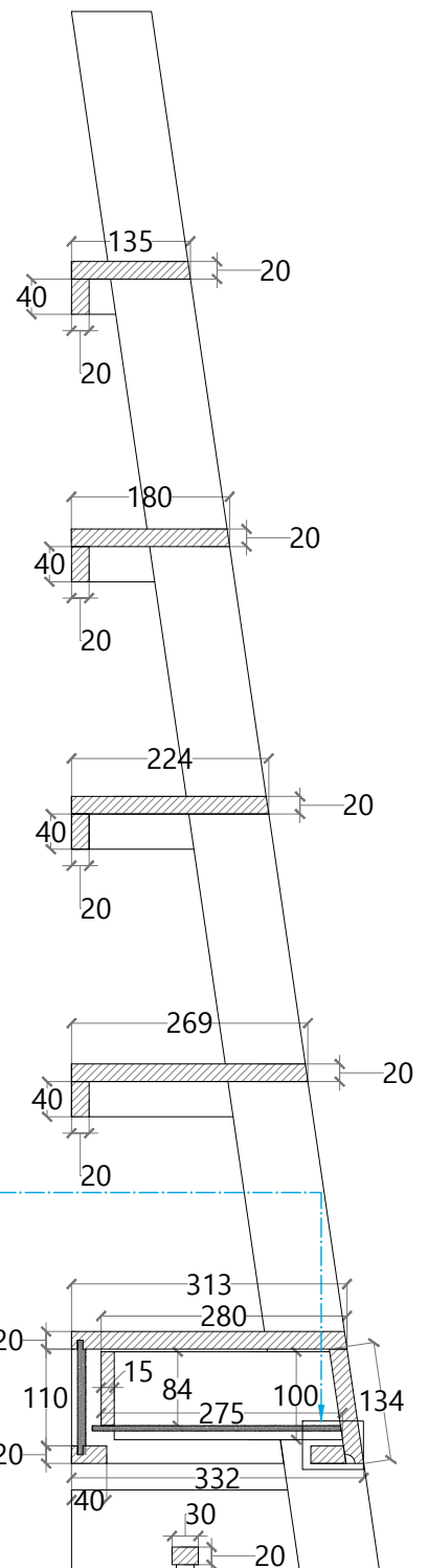
section B'
