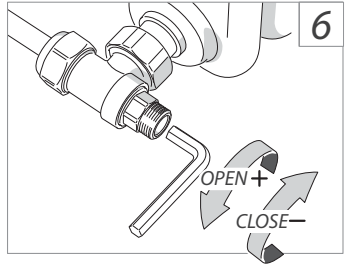
1/2" Art. 0223-0233
