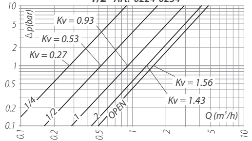
1/2" Art. 0224-0234
