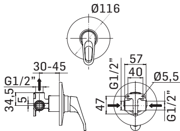
Gruppo monocomando da incasso per doccia ad 1 uscita Concealed 1-way single lever shower mixer
