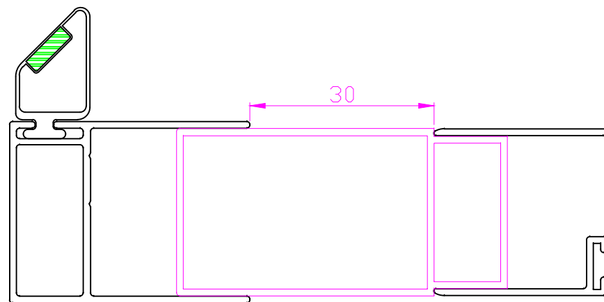
FA801 Door side
