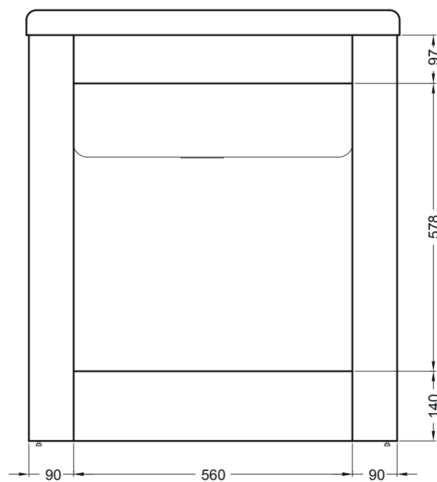
VISTA POSTERIORE
