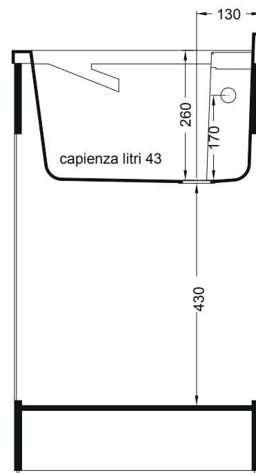
SEZIONE A-A
