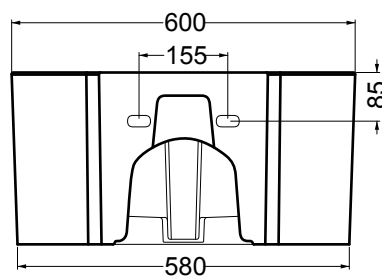
VISTA POSTERIORE
