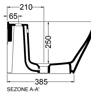
SEZIONE A-A'
