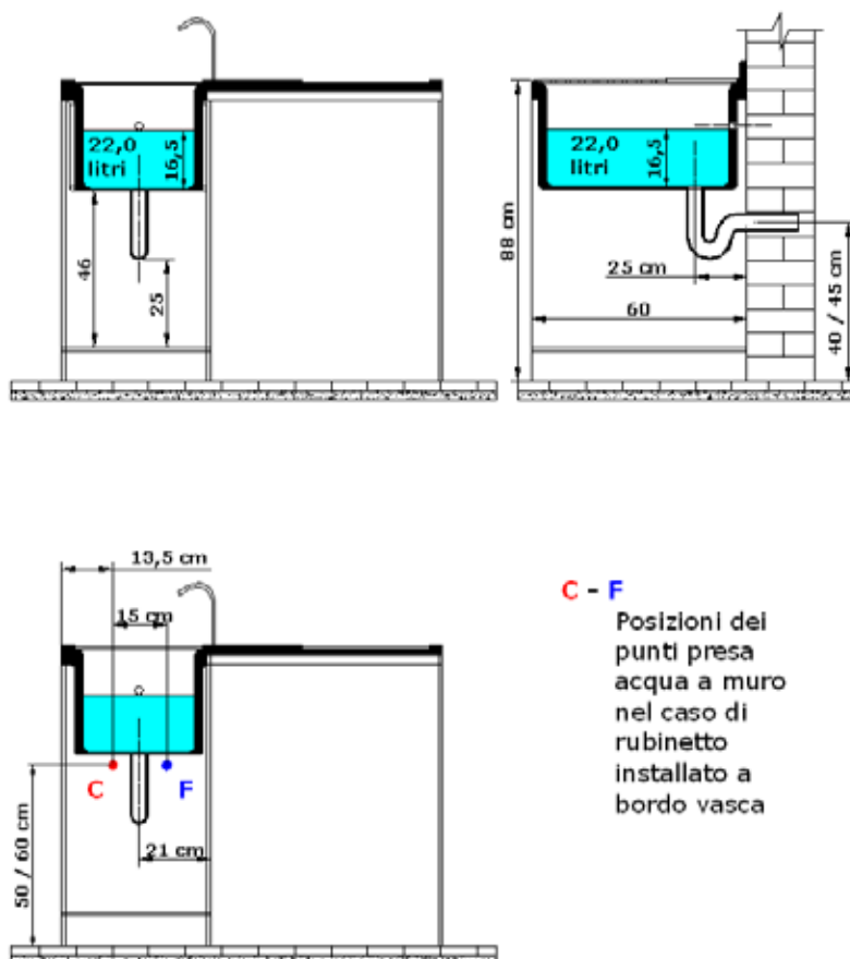
Posizionamento degli scarichi a muro
