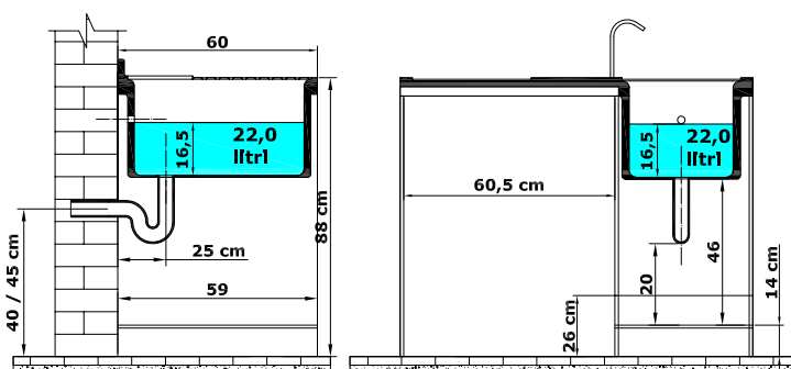
Posizionamento degli scarichi a muro
