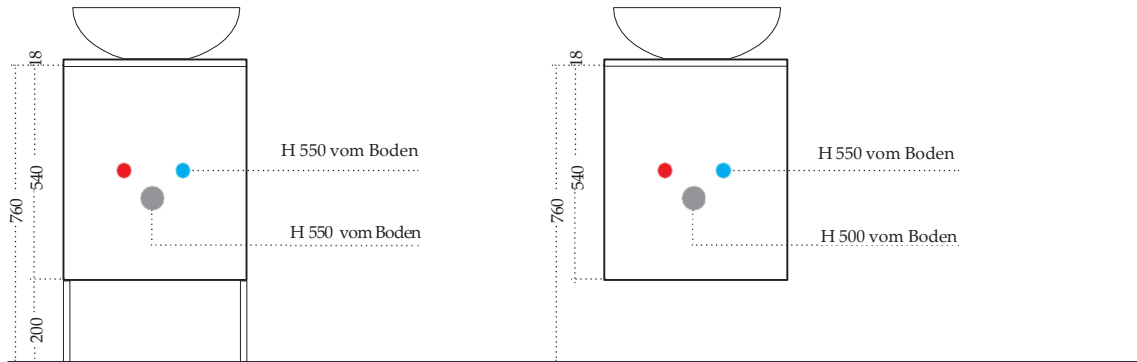
WASCHBECKENUNTERBAU 50 – MIT AUFSATZWASCHBECKEN
