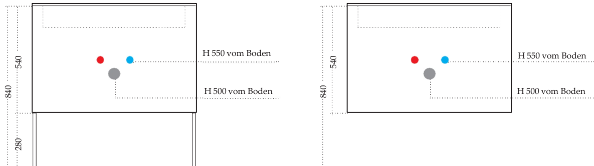
WASCHBECKENUNTERBAU 70 / 90 – mit integriertem oder halbeinbau-Waschbecken
